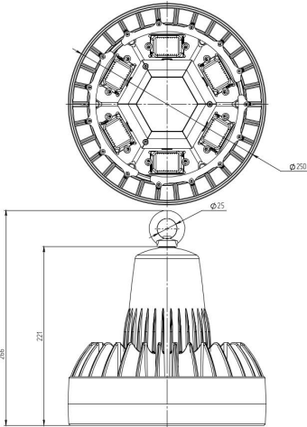
Рисунок 2. Габаритный чертеж
