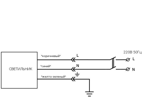
Рисунок 1. Электрическая схема подключения.
